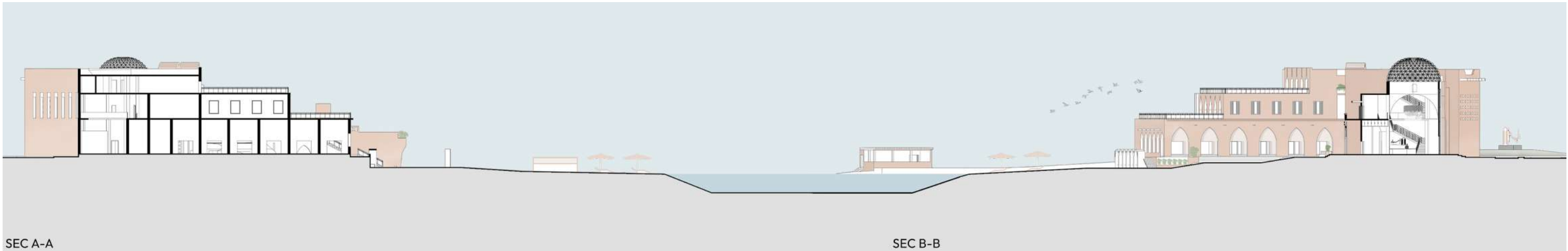
SEC A-A
